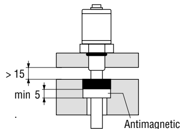
Alternative sealing O-Ring 15,3 x 2,2
